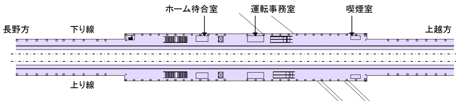
プラットホーム階 平面図
