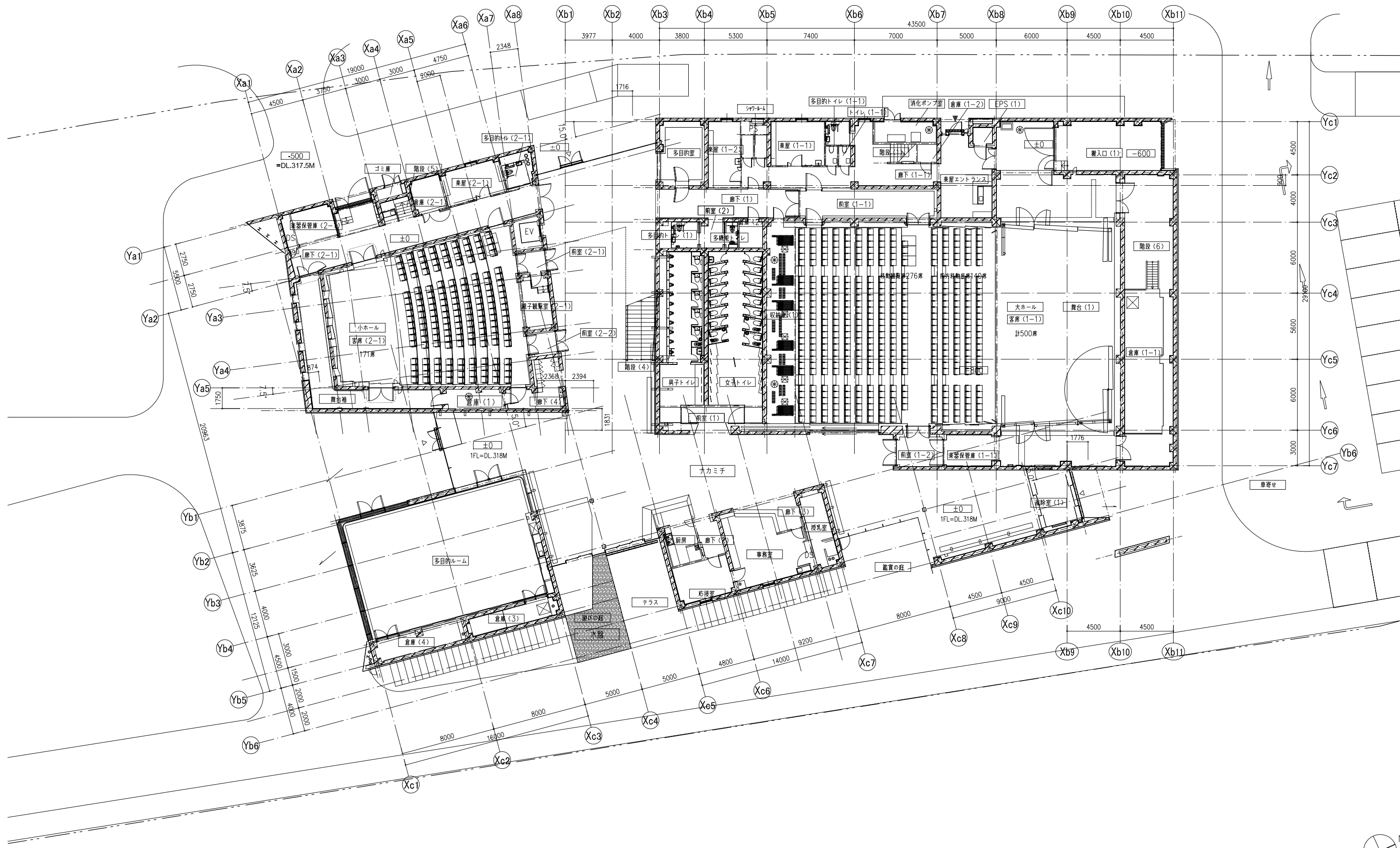
1階平面図
