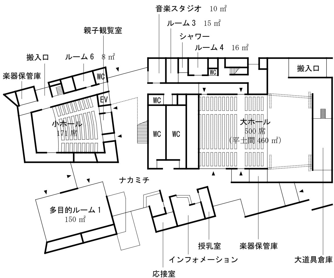
1F 平面図
