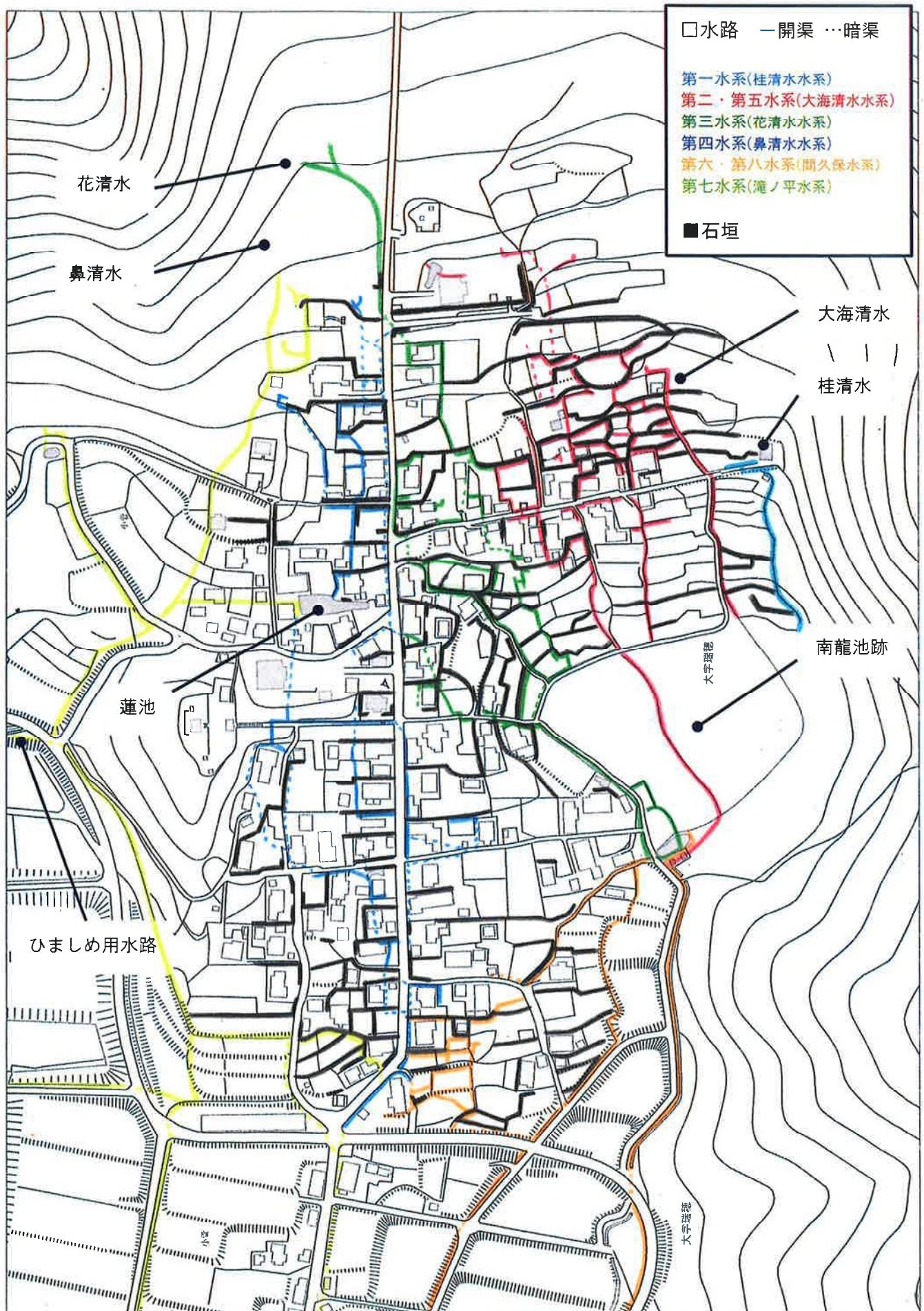
図7 集落内の石垣と水路の配置図
