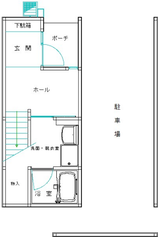
1階
