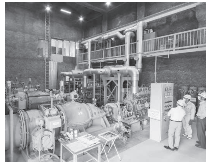
▲復旧したポンプ室内部
