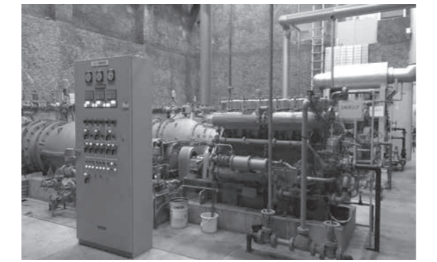
機械設備更新中のポンプ室内部
