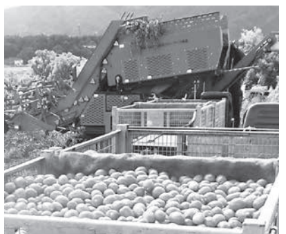
▲ジュース用トマト専用収穫機
