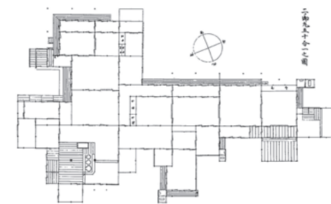
二の丸御殿平面図
