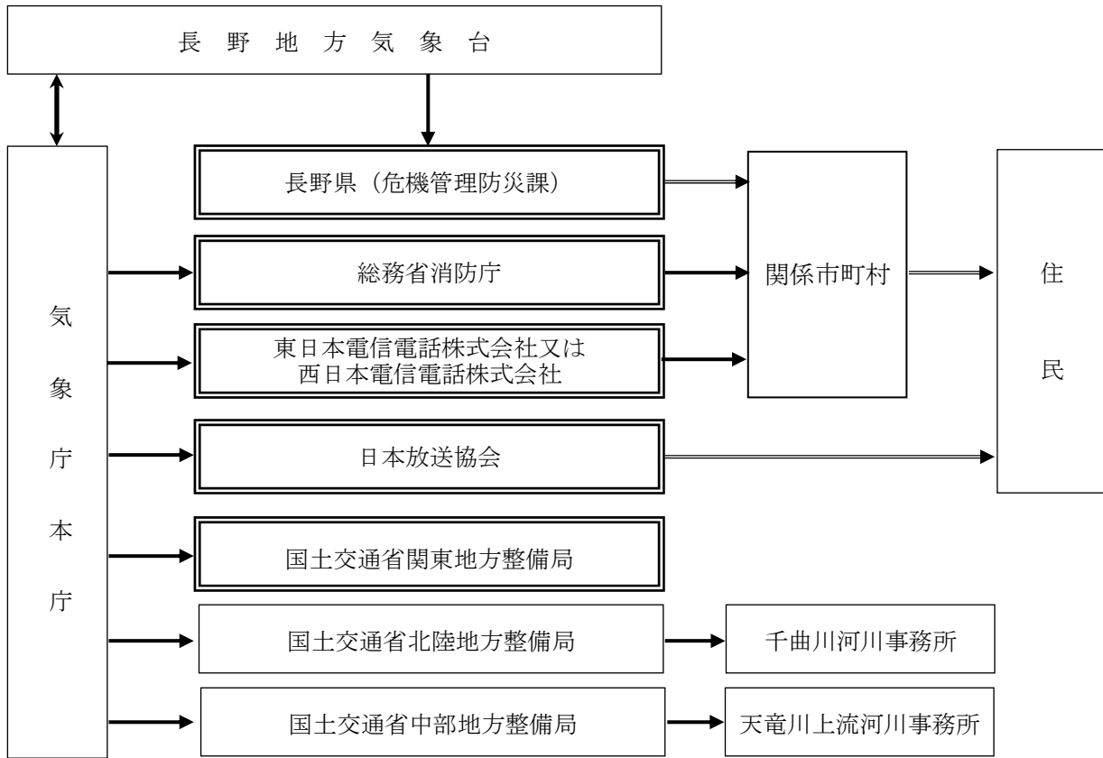
伝達系統図
