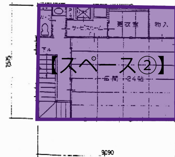
2階平面図 95.30㎡(土蔵 26.44㎡)
